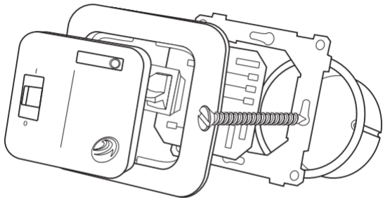
Рис.3 Установка контроллера СКПВ220В-мини2N в распаечную коробку
