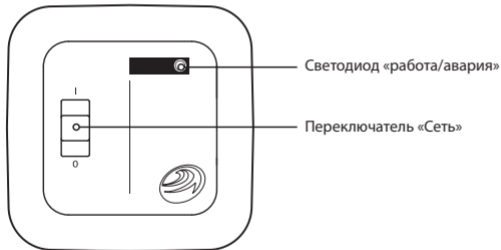
Рис.1 Контроллер СКПВ220В-мини2N
